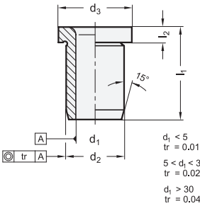
DIN 172-ST
